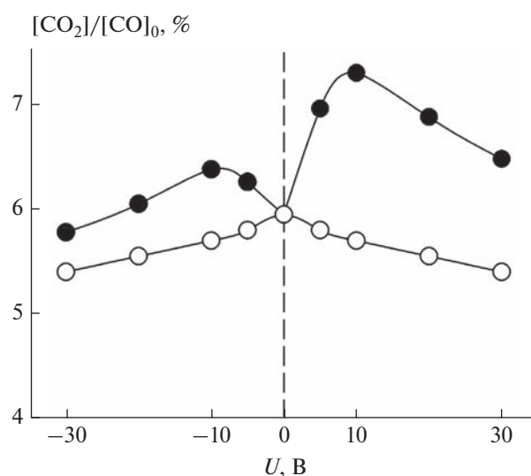
Рис. 1. Конверсия СО на покрытии из наночастиц золота при различных напряжениях, подаваемых на покрытие. Черные точки — конверсия при последовательной подаче положительных и отрицательных напряжений, светлые — конверсия при U = 0 как до, так и после подачи напряжения.
