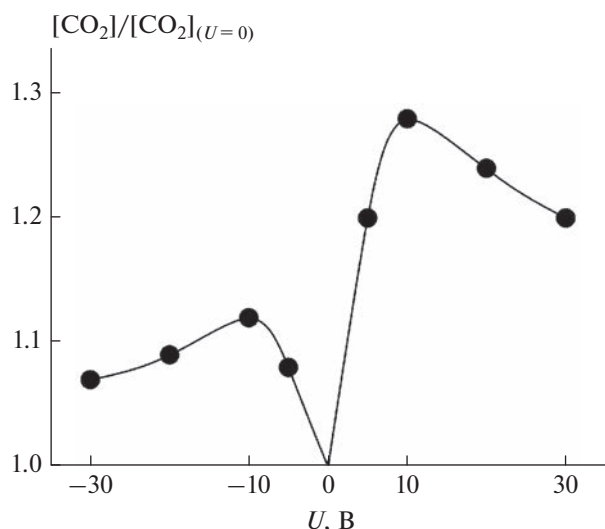
Рис. 2. Увеличение конверсии СО на покрытии из наночастиц золота при последовательном увеличении подаваемого на покрытие положительного или отрицательного напряжения.
