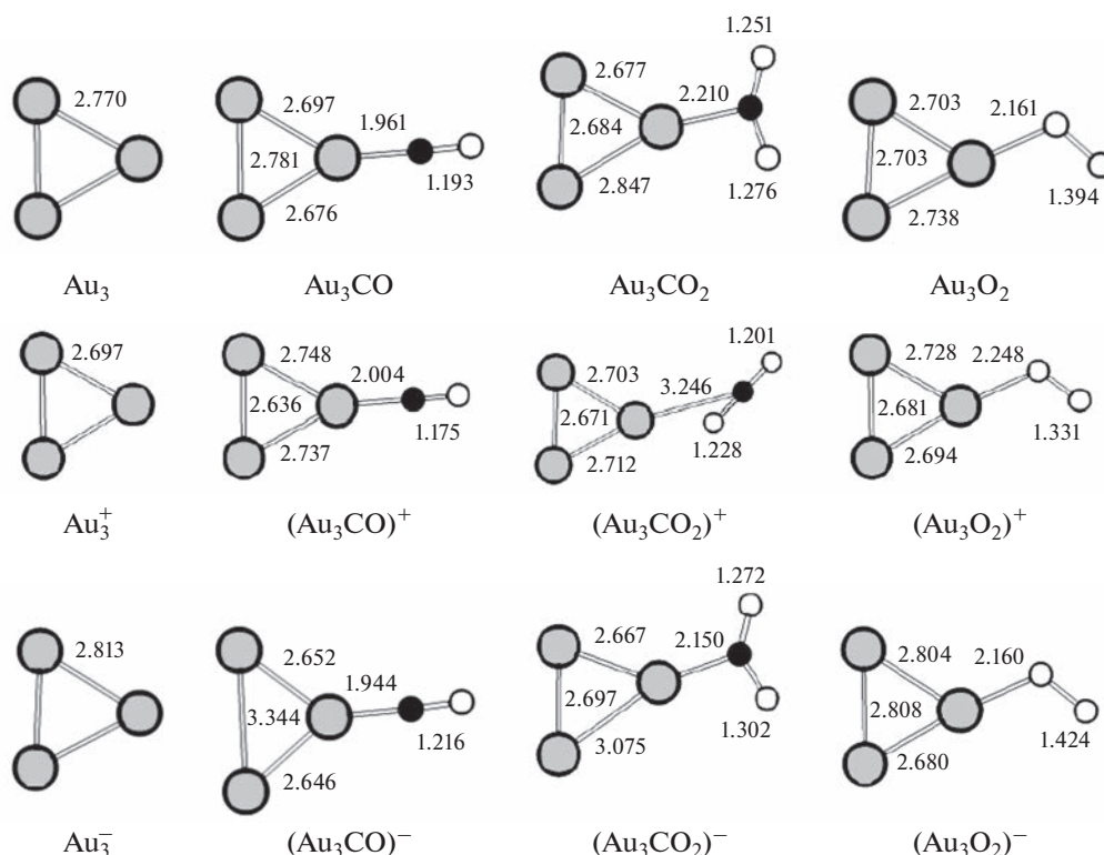
Рис. 3. Структуры электронейтральных, а также положительно и отрицательно заряженных \text{Au}_3 -содержащих соединений: серые кружки — Au, черные — C, белые — O. Числа — расстояния в Å.
